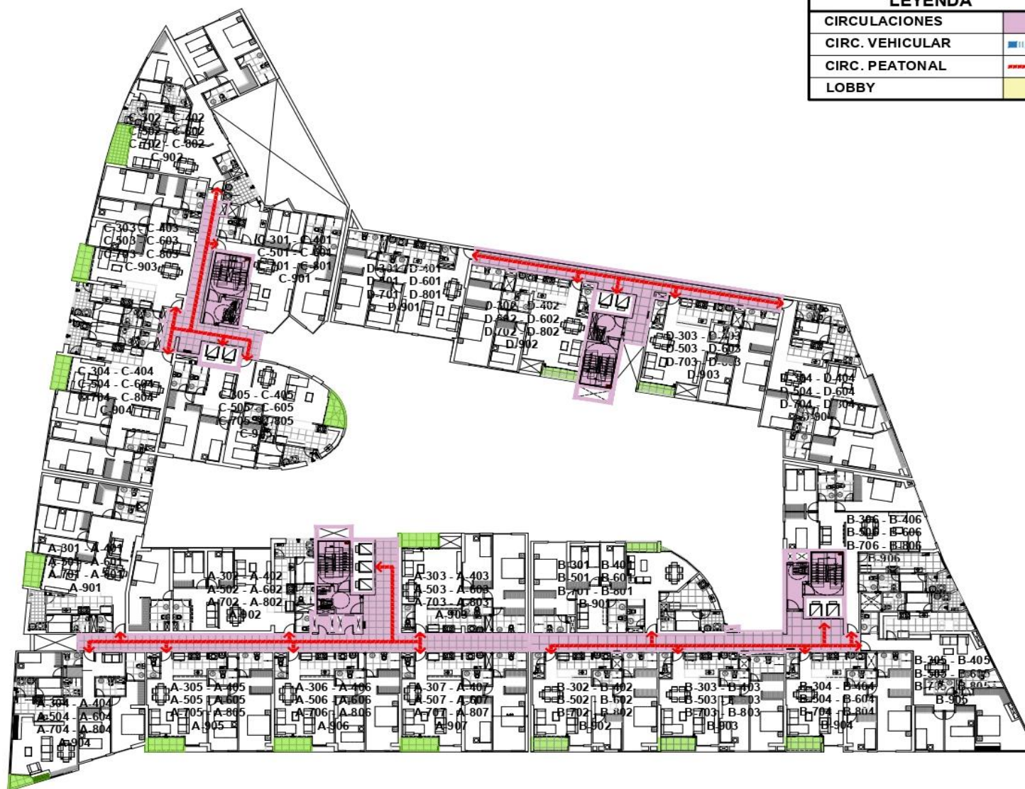
PLANTA TIPICA
